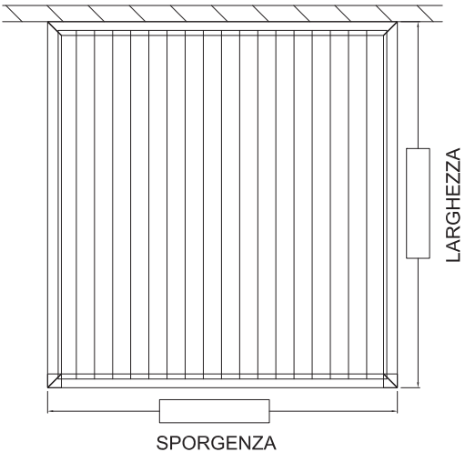
Lame perpendicolari al muro
