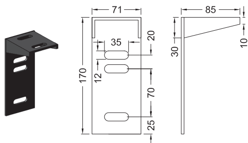
piastra ancoraggio a soffitto € 94,00 pz
