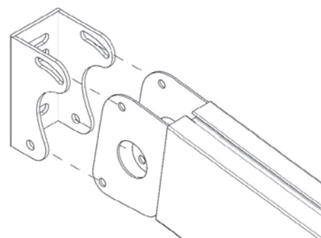
attacco a parete
