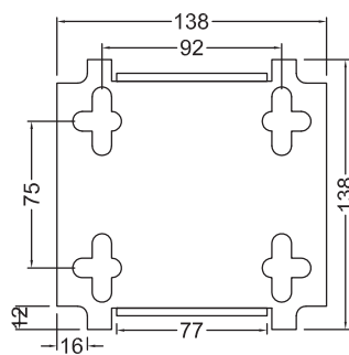
staffa piantana
