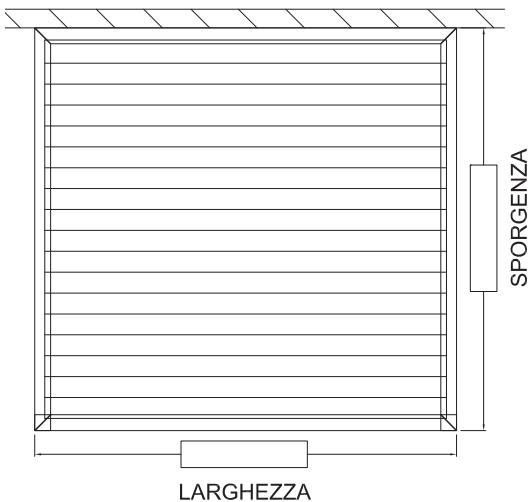
Lame parallele muro
