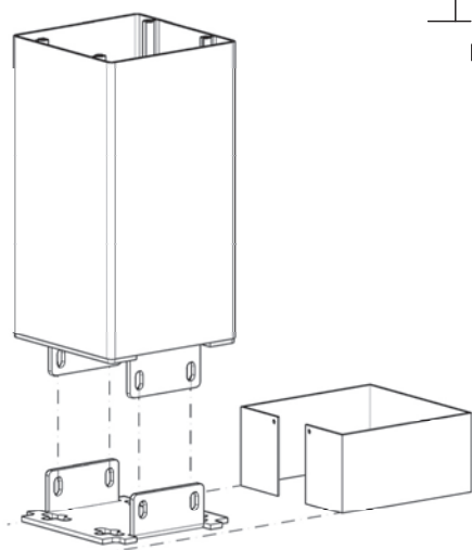
attacco a pavimento
